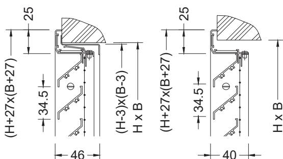
Type ACQXAR. (INCL. INBOUWRAAM)
