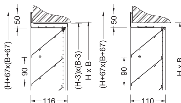
Type ACPZAR. (INCL. INBOUWRAAM)
