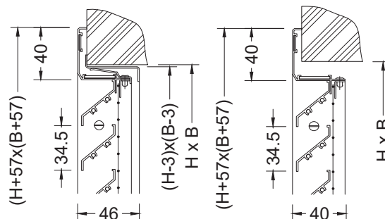
Type ACQYAR. (INCL. INBOUWRAAM)
