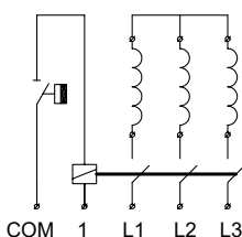
Aansluitschema 1-traps, 400V/3ph
