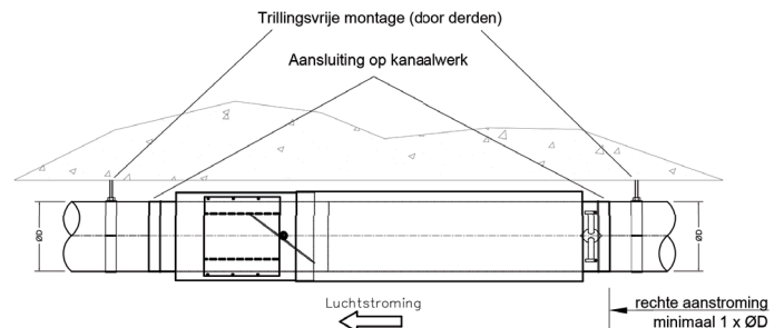
Montagetekening type NBOEORB (retour)
