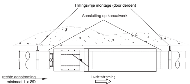
Montagetekening type NBOEOB (toevoer)
