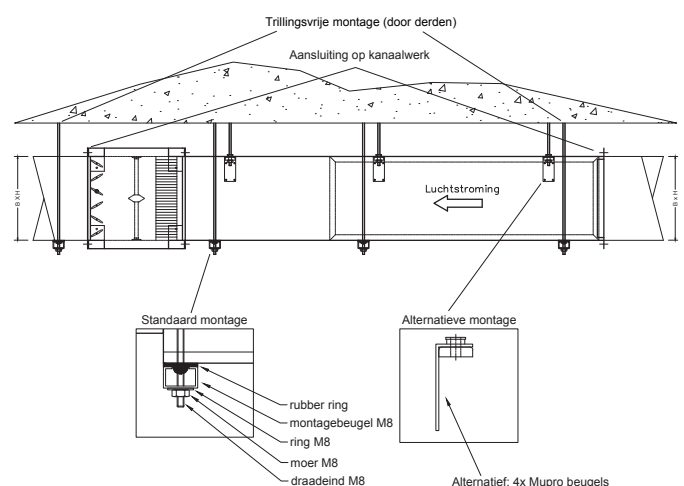
Montagetekening type NLOFORB (retour variant)
