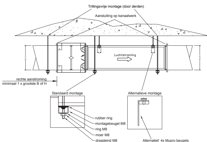
Montagetekening type NLOFOOB (toevoer variant)
